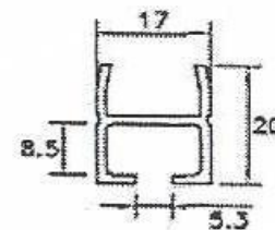
DETALLE - 2
